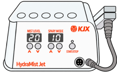
②噴槍與主機連接4Pin線
